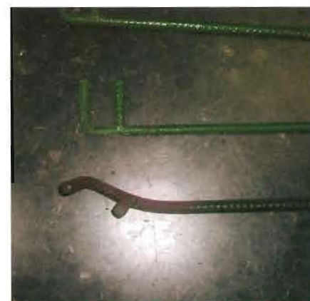
Figura 2. Útil doblado por efecto de la fatiga
